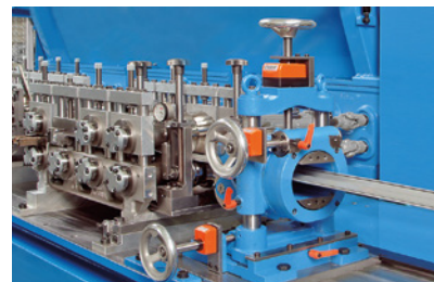
Regolazione precisa delle macchine per la lavorazione della lamiera
